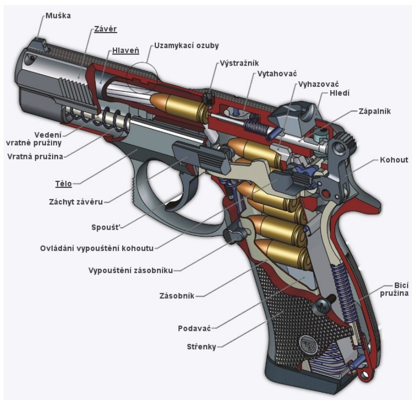
Obrázek 2. Popis hlavních částí a ovládacích prvků pistole [10]
