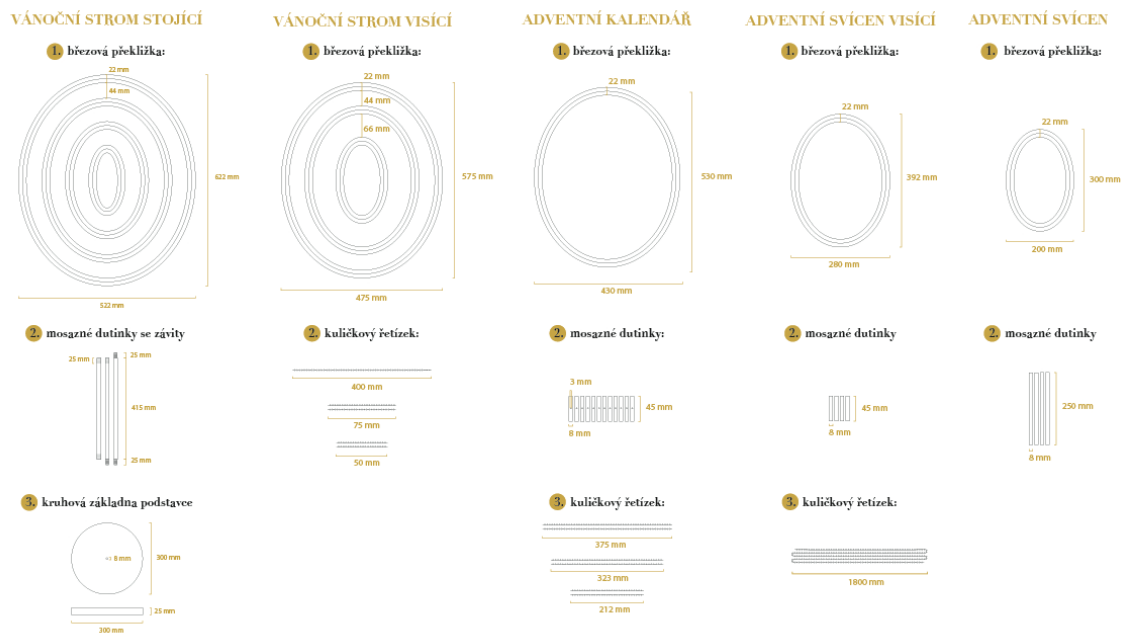
Obr. 188 Rozměry jednotlivých komponentů
